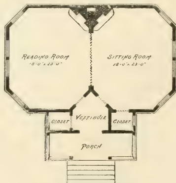
FIG. 95.—GROUND-PLAN.
