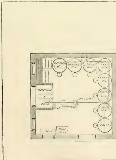
FIG. 212.—GROUND-PLAN.
