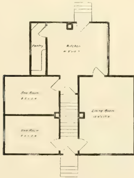
FIG. 86.—GROUND-PLAN.
