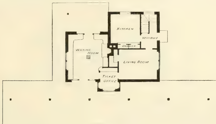
FIG. 500.—GROUND-PLAN.
