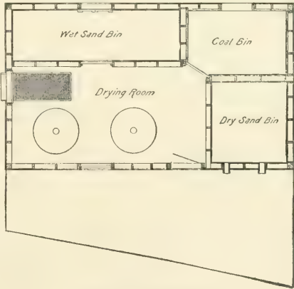
FIG. 178.—GROUND-PLAN.
