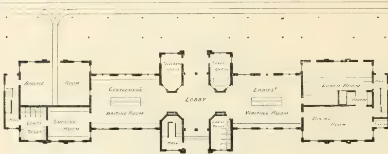
FIG. 561.—GROUND-PLAN.
