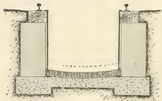
FIG. 146.—CROSS-SECTION
