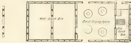
FIG. 179.—GROUND-PLAN.
