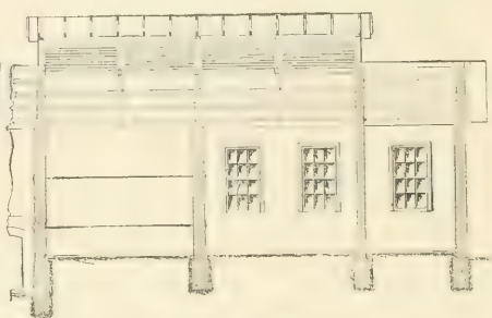
FIG. 186. LONGITUDINAL SECTION.
