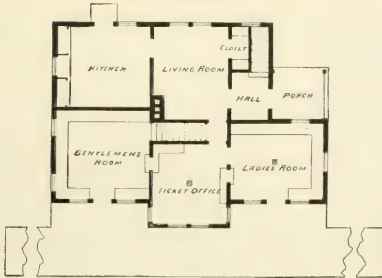
FIG. 494.—GROUND-PLAN.
