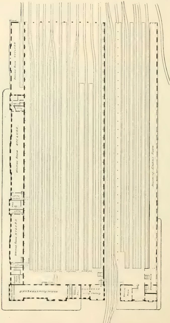
FIG. 673.—GROUND-PLAN.
