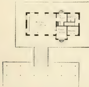
FIG. 553.—GROUND-PLAN.
