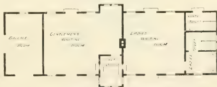
FIG. 517.—GROUND-PLAN.
