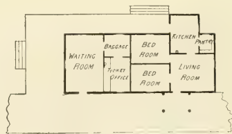
FIG. 504.—GROUND-PLAN.
