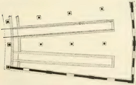
FIG. 330.—GROUND-PLAN.
