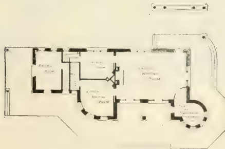
FIG. 560.—GROUND PLAN.
