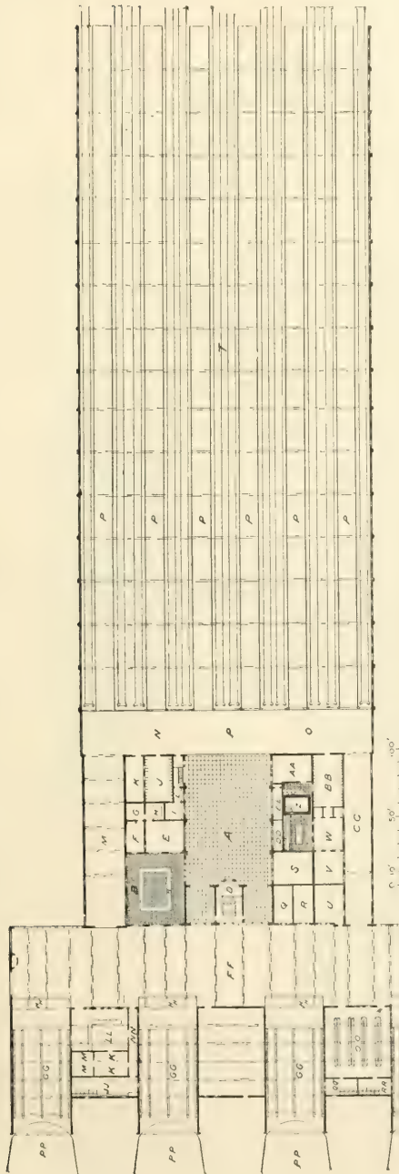
FIG. 679.—GROUND-PLAN.
