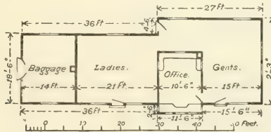
FIG. 570.—GROUND-PLAN.
