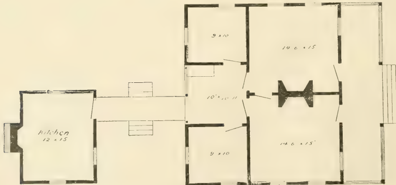
FIG. 63.—GROUND-PLAN
