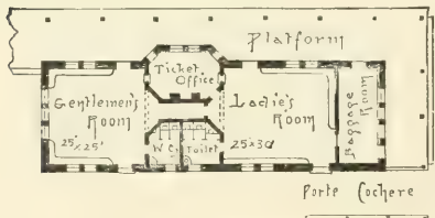
FIG. 595.—GROUND-PLAN.
