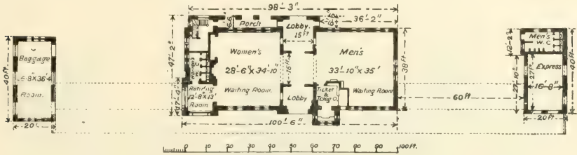
FIG. 566.—GROUND-PLAN.
