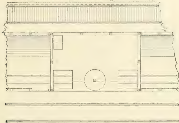
FIG. 271.—GROUND-PLAN.
