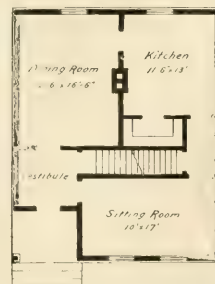
FIG. 84.—GROUND-PLAN.
