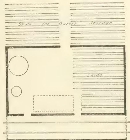
FIG. 223.--GROUND PLAN.
