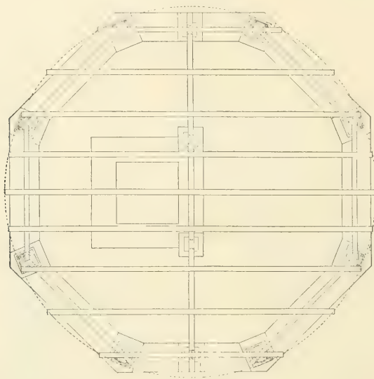
FIG. 266.—GROUND-PLAN.
