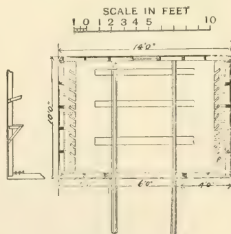
FIG. 35.—GROUND-PLAN.
