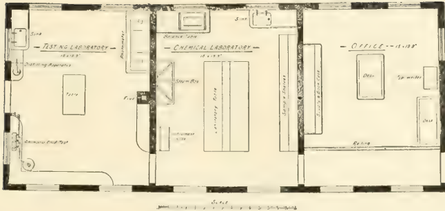
FIG. 239.—GROUND PLAN.
