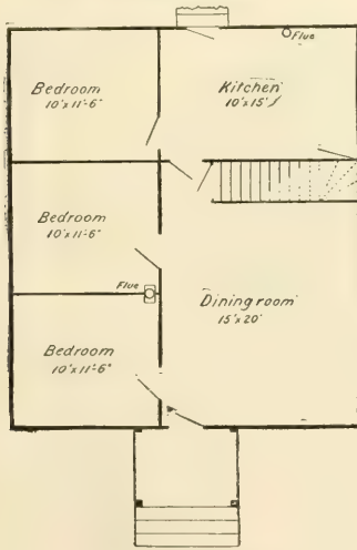
FIG. 59.—GROUND-PLAN.
