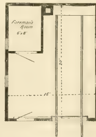
FIG. 39. GROUND-PLAN.
