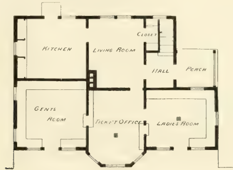
FIG. 506.—GROUND-PLAN.
