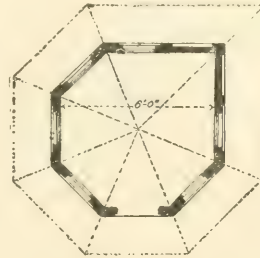
FIG. 5.—GROUND-PLAN.
