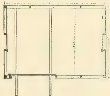
FIG. 24.—GROUND-PLAN.
