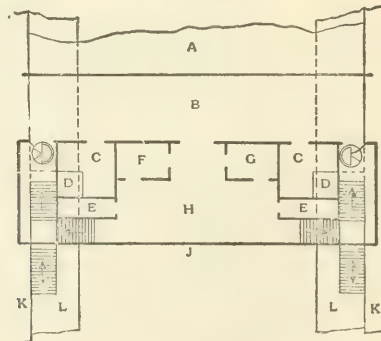
FIG. 581.—GROUND-PLAN.
