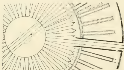
FIG. 324.—GENERAL PLAN.
