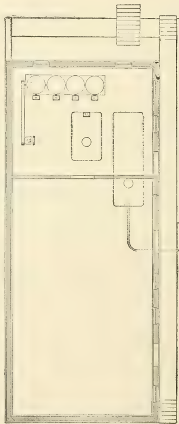
FIG. 220.—GROUND-PLAN.
