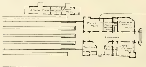
FIG. 642.—GROUND-PLAN.
